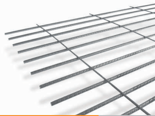
Ø12/200mm
